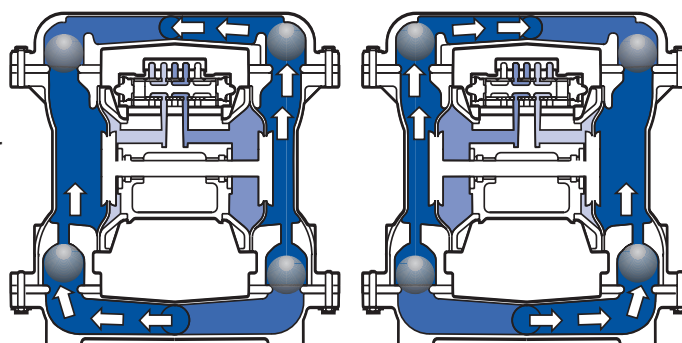
Right chamber—discharge
